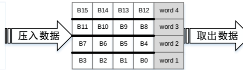
图 10-4. PWIDTH 为‘0b00’时，数据的打包 / 解包
