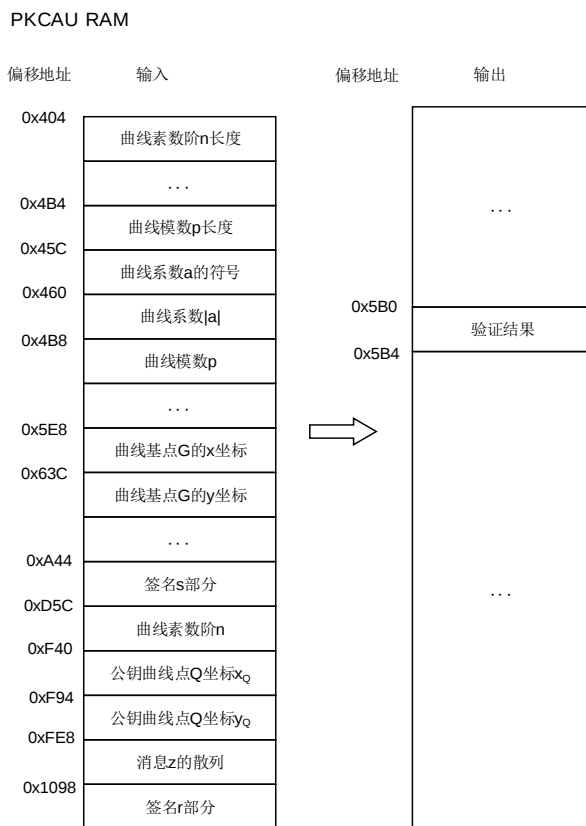
图 22-23. ECDSA 验证
