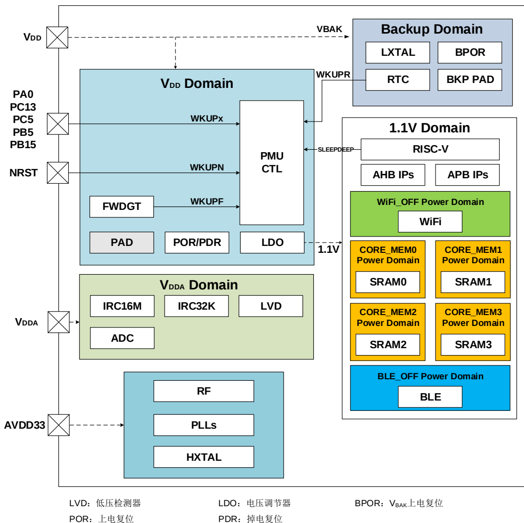
图 4-1. 电源域概览
