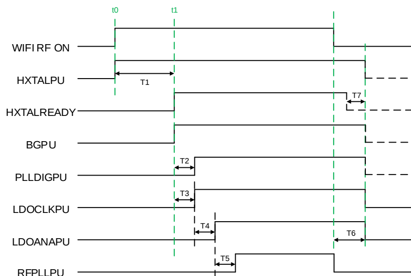
图 4-4. RF 时序
