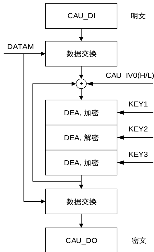
图 20-6. DES / TDES CBC 加密
