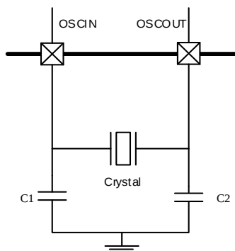
图 5-3. HXTAL 时钟源
