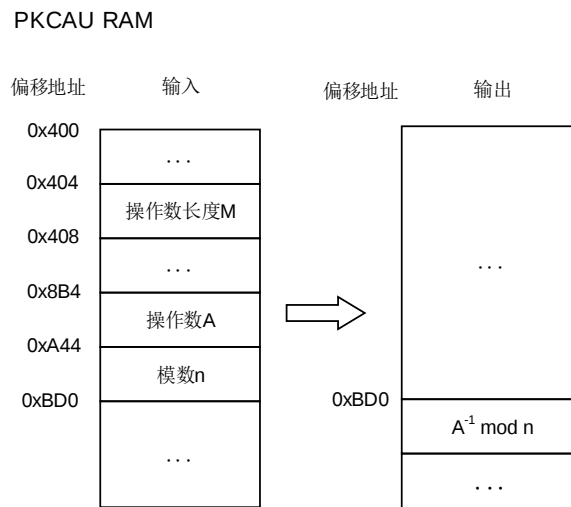
图 22-17. 模逆运算
