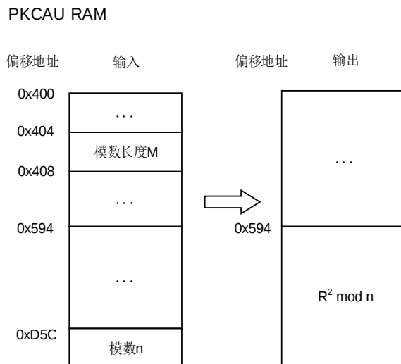
图 22-12. 蒙哥马利参数计算
